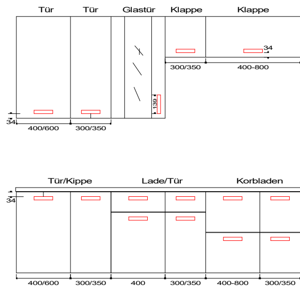
BOHRBILD: BM374
