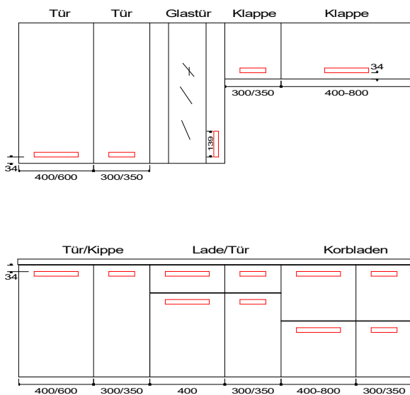
BOHRBILD: BM27
